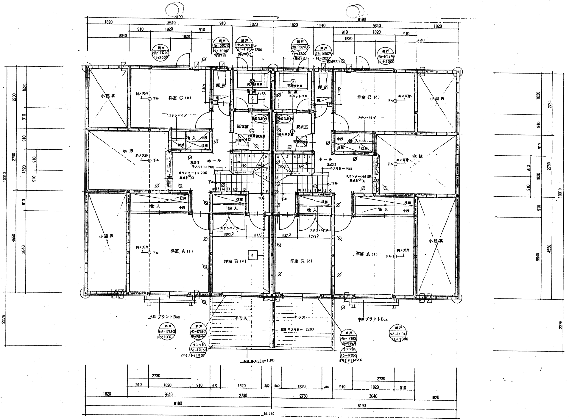
2階平面図
