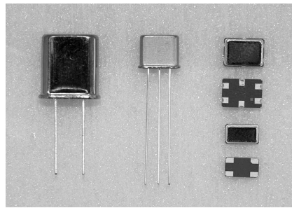
▲ソラチ・クォーツで生産されている精密な電子部品。
